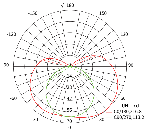
配光曲线
